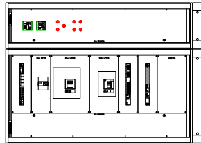
QUADRO GENERALE BANCA TENSIONE GGBT TR1 - ESISTENTE
